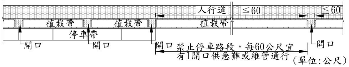
圖 13.2.1 綠帶間設置開口原則參考圖
